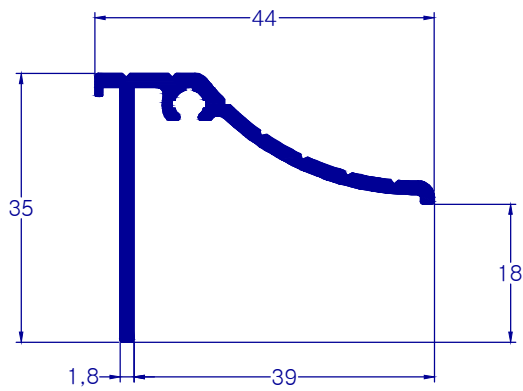
CM-169 0,431 kg/m
