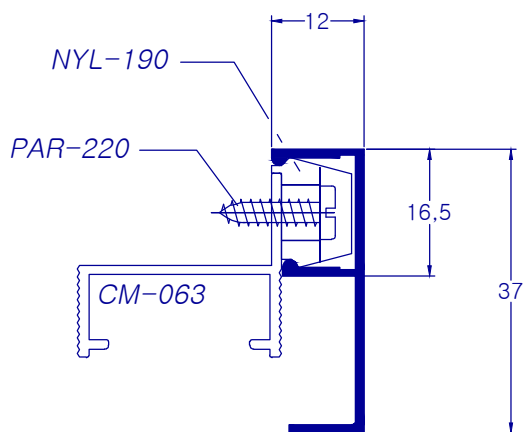
MP-347 0,202 kg/m
