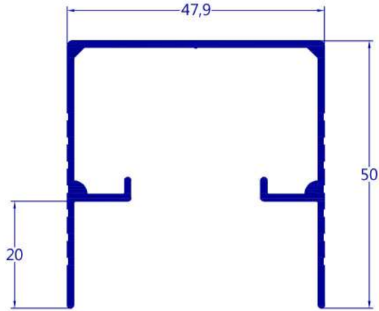
U-655 BX-183 0,591 kg/m
