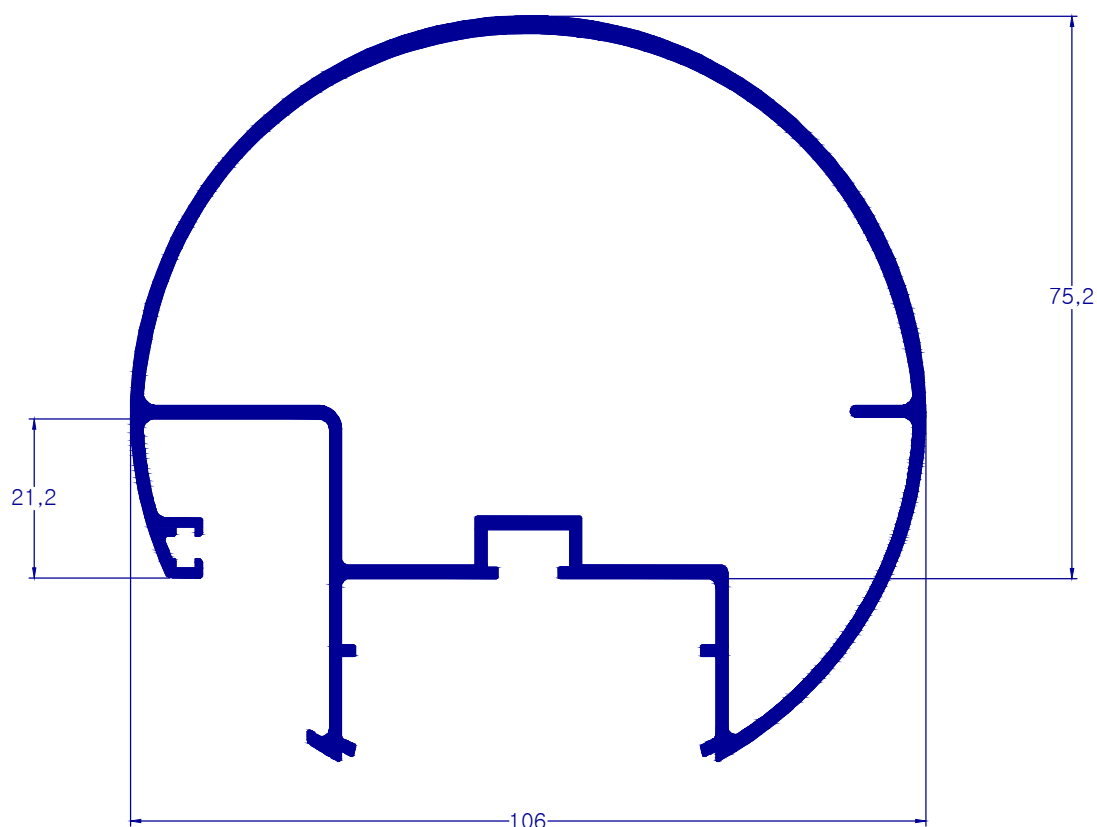
D-201* 1,899 kg/m
