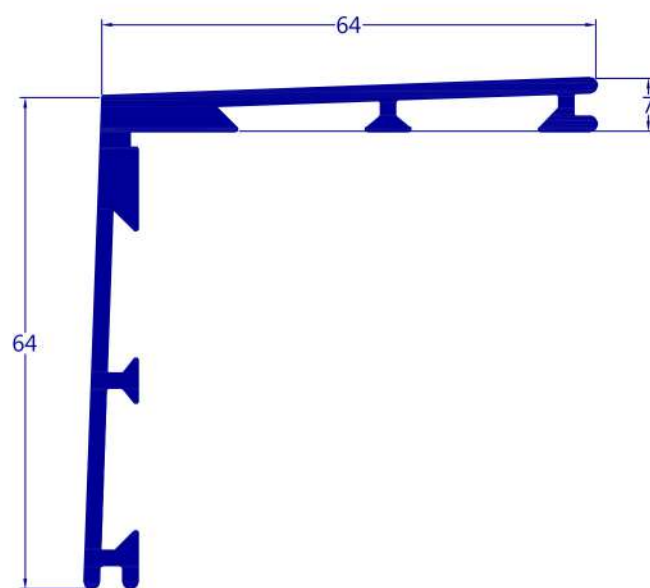
L-579 CL-044 1,080 kg/m
