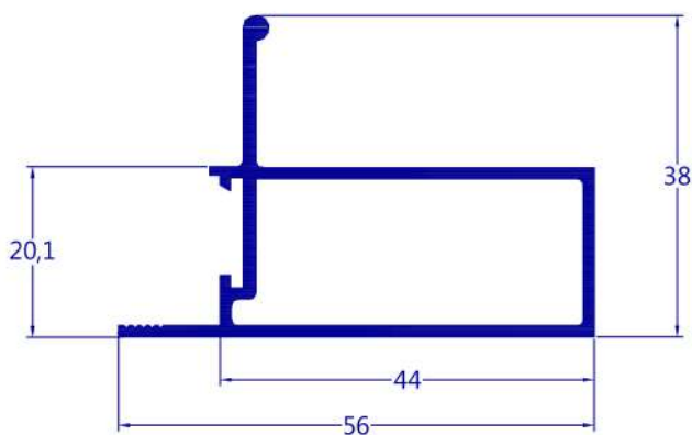
MP-337 0,585 kg/m
