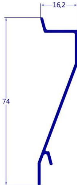
VZ-023 0,292 kg/m
