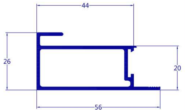
MP-070 0,599 kg/m
