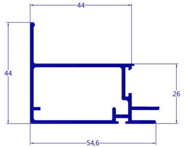
MP-069 0,728 kg/m
