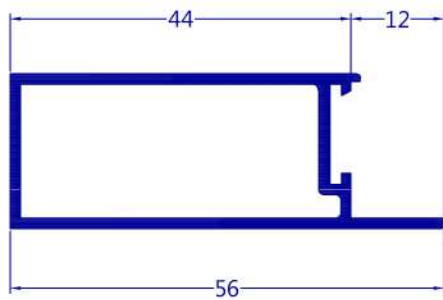
MP-336 0,499 kg/m
