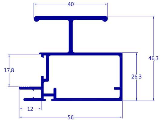
MP-379 0,978 kg/m
