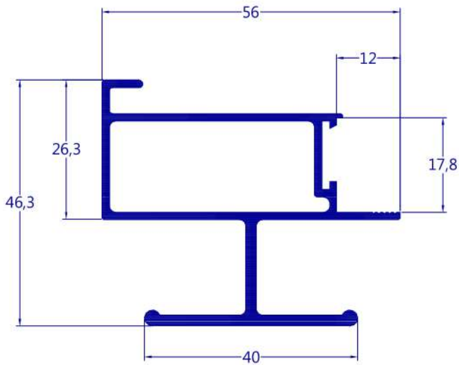
MP-380 0,905 kg/m
