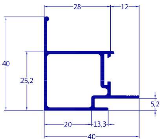
MP-300 0,370 kg/m
