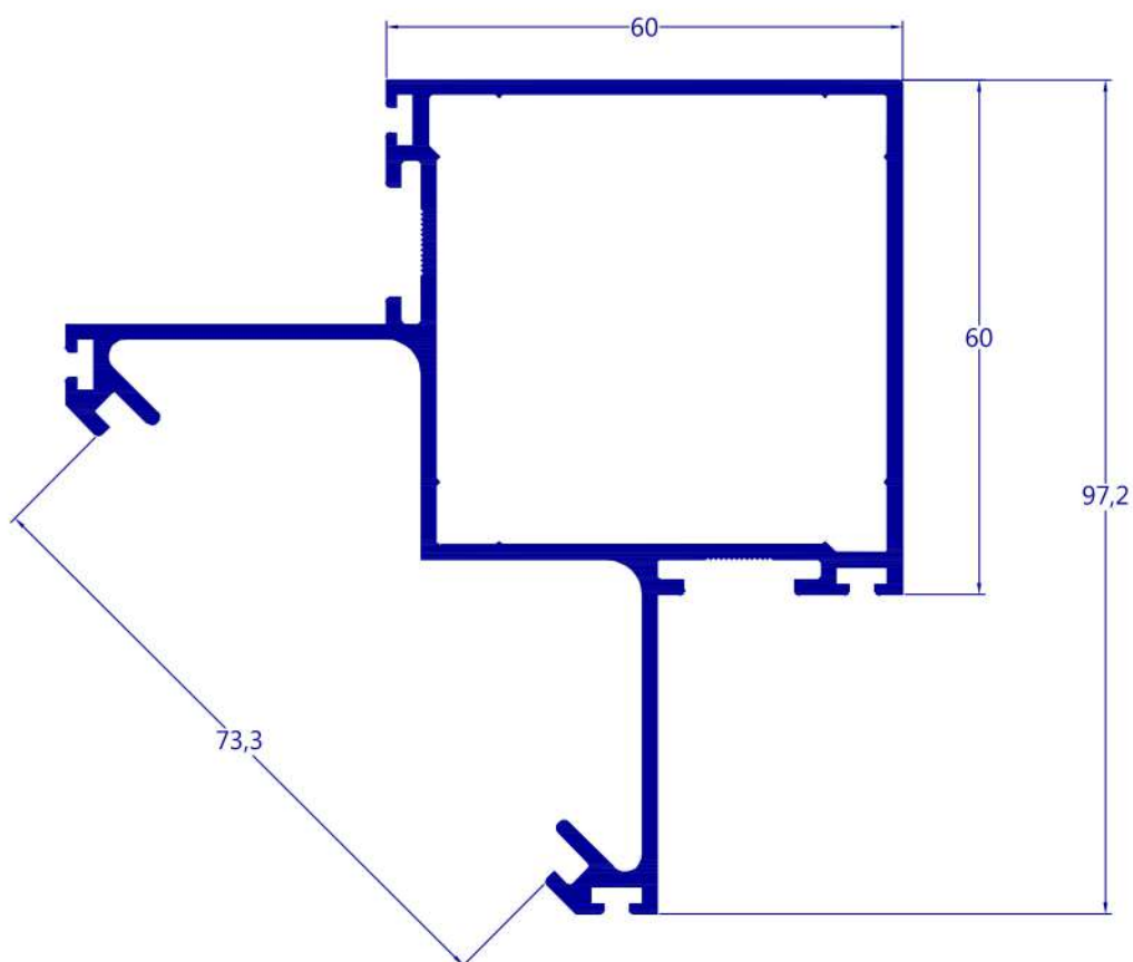
FC-244 1,786 kg/m
