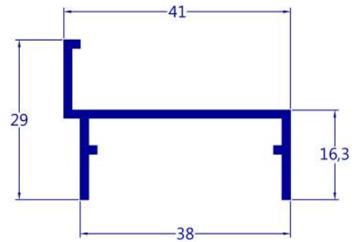
PC-007 0,358 kg/m
