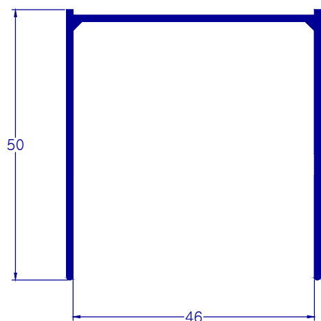
U-599 0,593 kg/m
