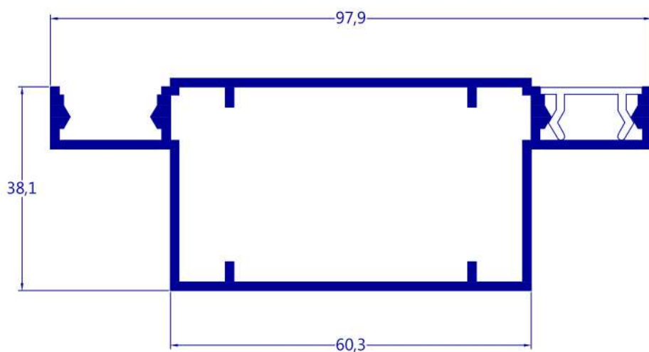
D-777 0,974 kg/m
